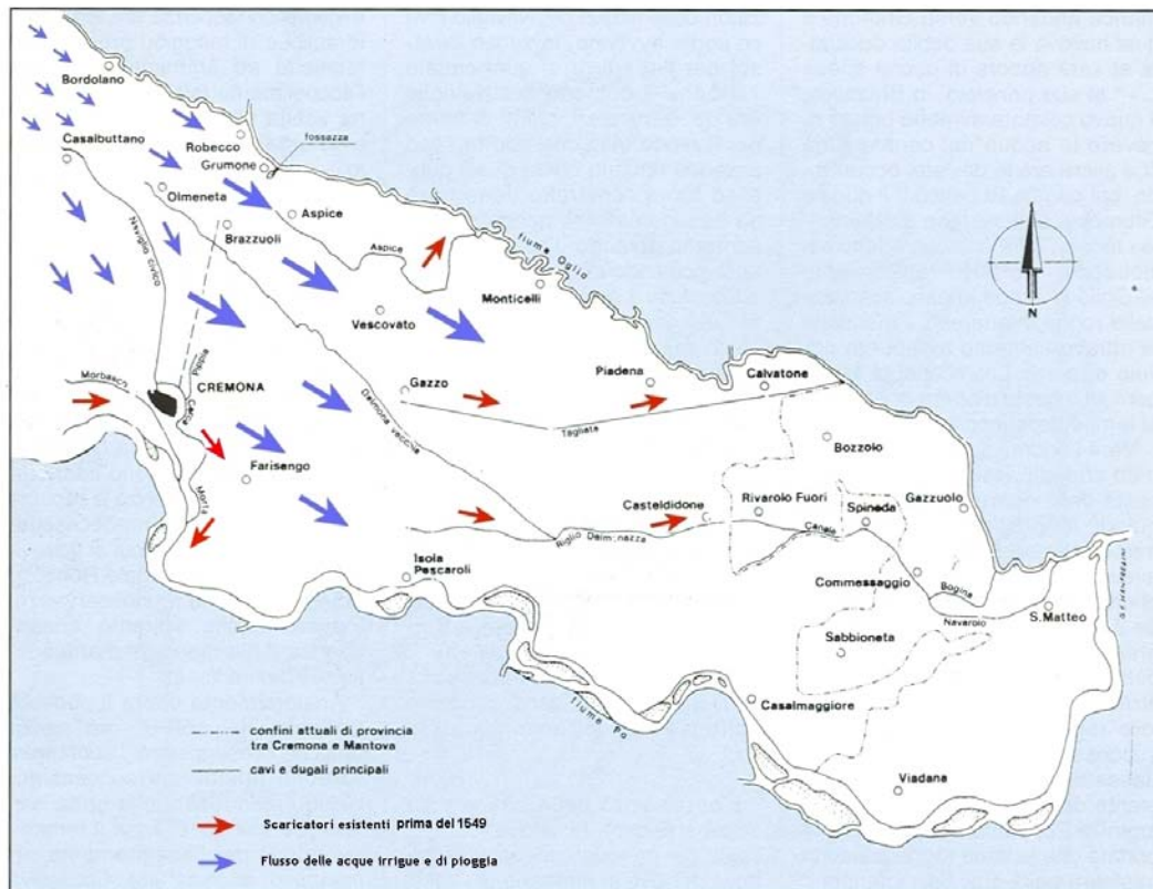
Flusso delle acque sul territorio a Nord di Cremona prima della realizzazione del Dugale di Robecco (1549).
