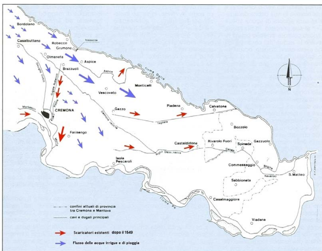
Direzione delle acque nel territorio cremonese dopo la realizzazione del Dugale di Robecco: è evidente la funzione di "trincea idraulica" svolta dal nuovo cavo che ha ridotto drasticamente le portate prima dirette verso le terre basse ad oriente di Cremona.
